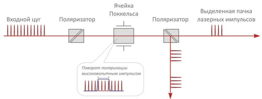
Оптический блок селектора OG-V для Yb фс лазера
